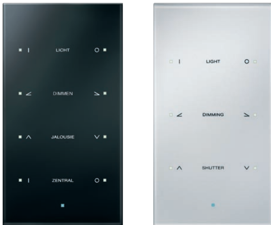
Berker TS Sensor in Schwarz, Alu und Polarweiß (rechte Seite) mit Beschriftung und Symbolik
